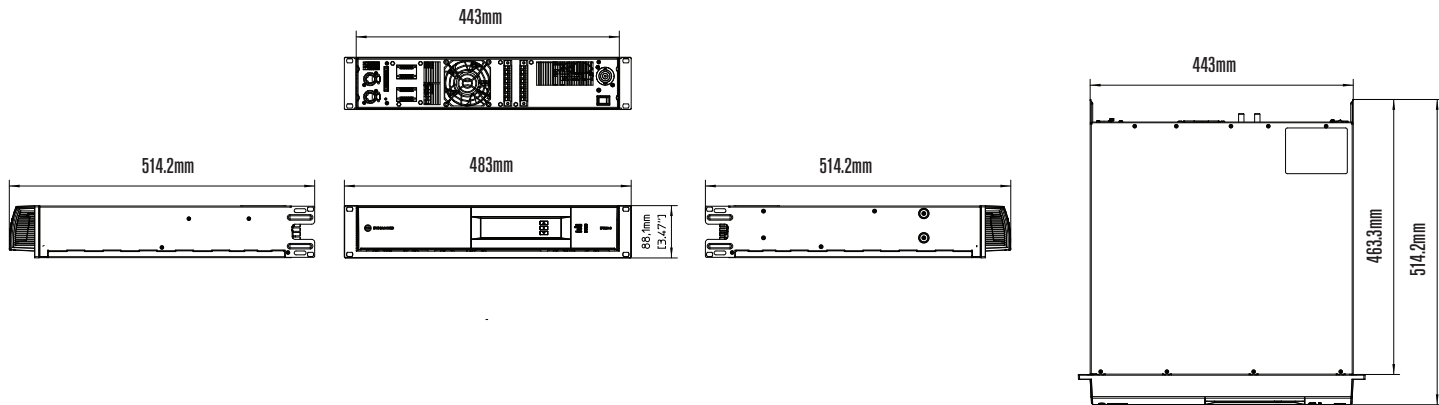
寸法図
