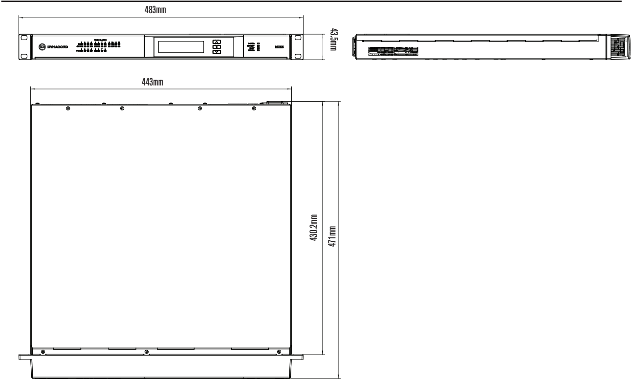
寸法図
