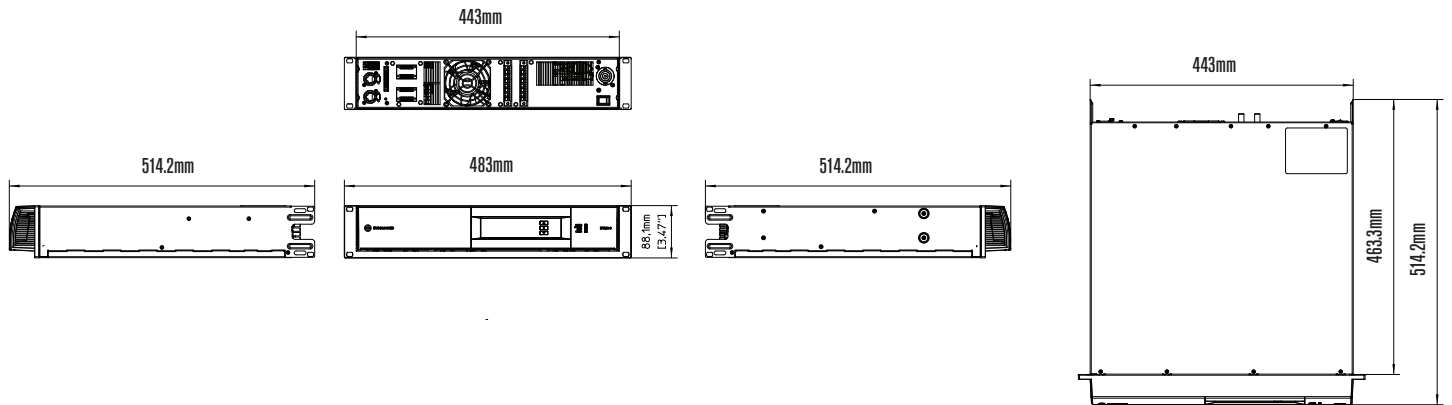
寸法図
